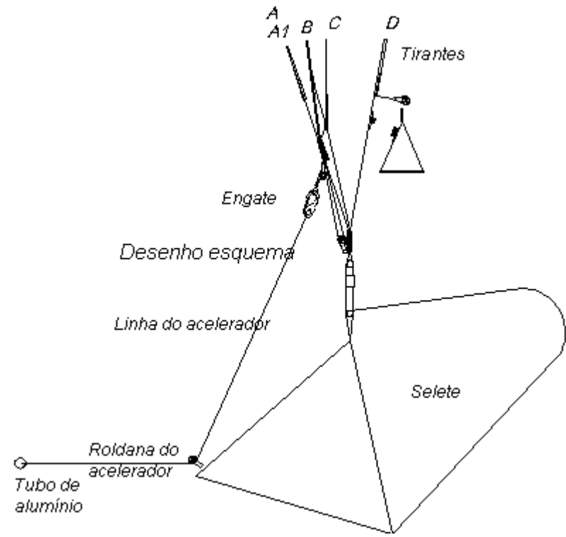
Desenho detalhe
